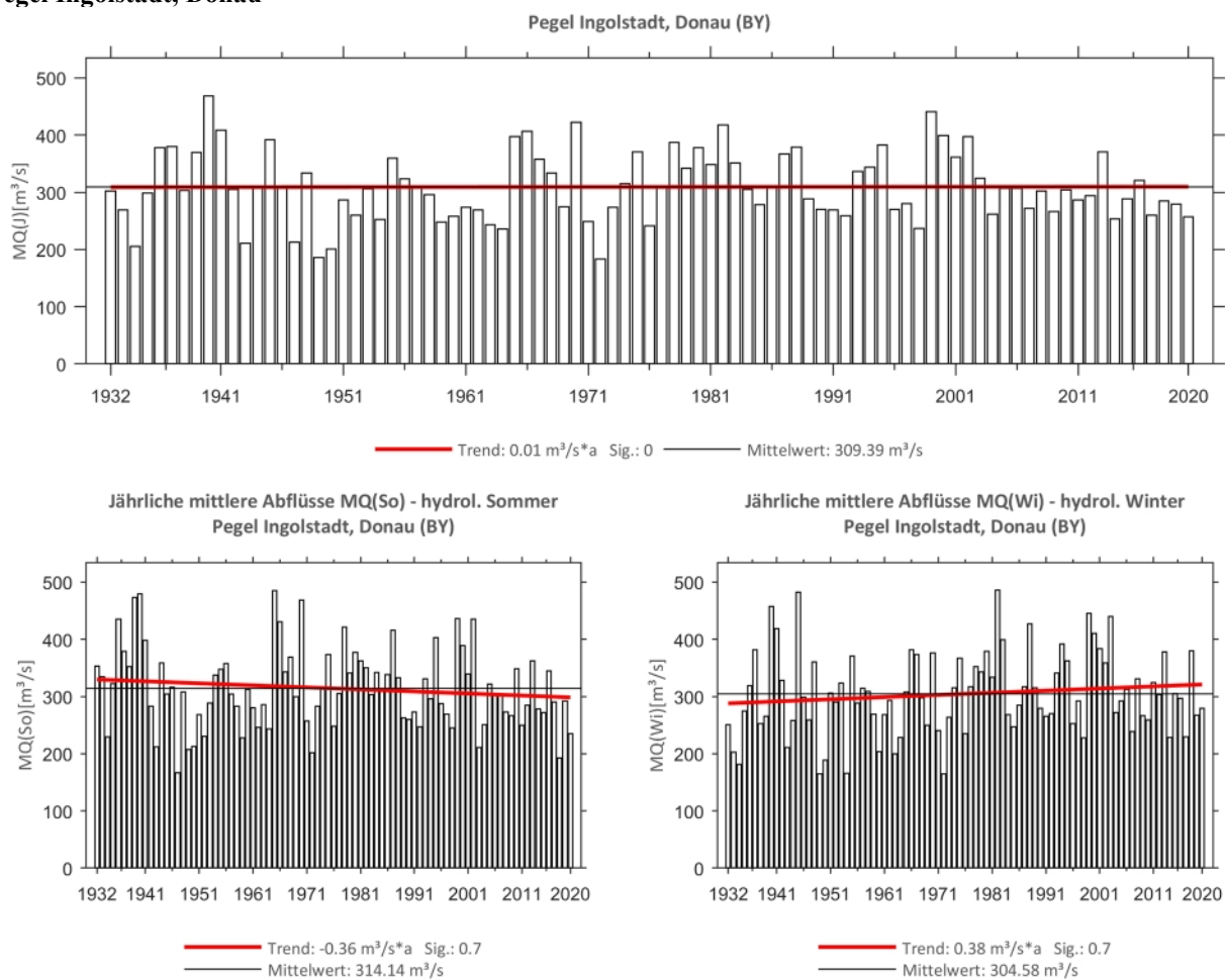
Abb. 142: Trenduntersuchungen von jährlichen mittleren Abflüssen für den Zeitraum 1932 bis 2020.
