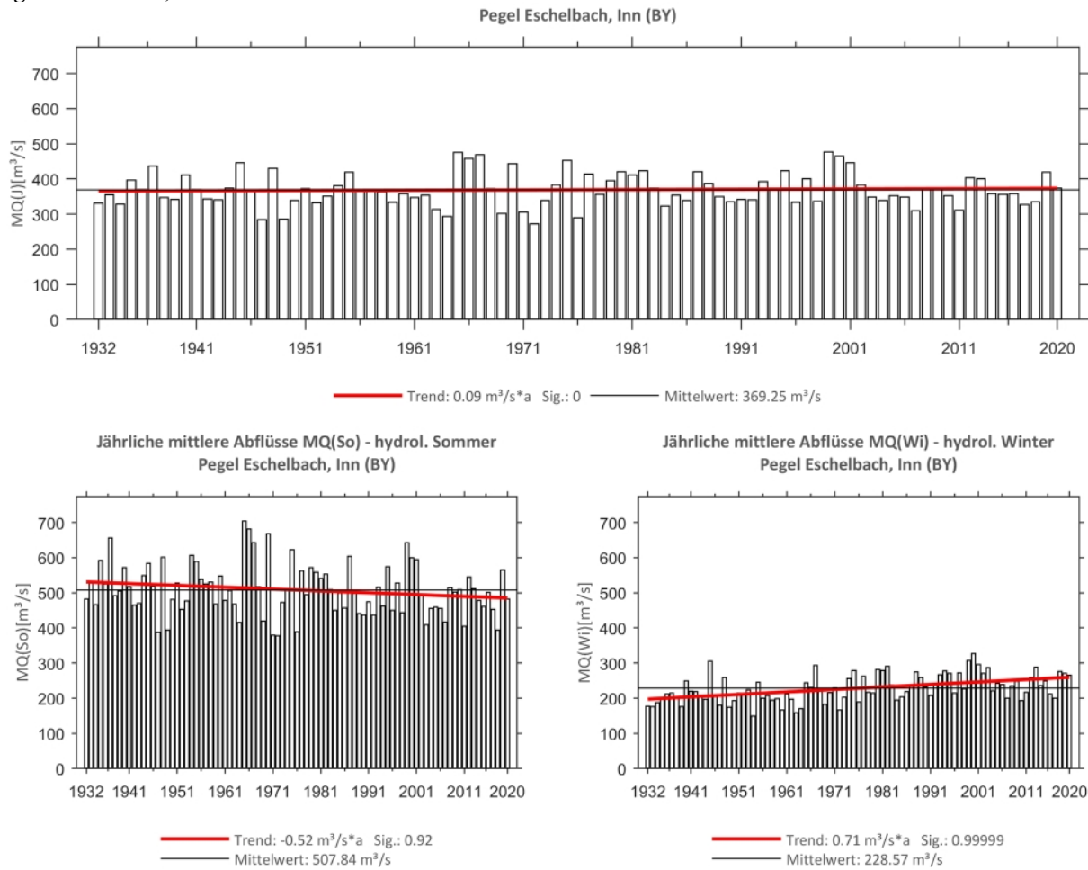
Abb. 106: Trenduntersuchungen von jährlichen mittleren Abflüssen für den Zeitraum 1932 bis 2020.
