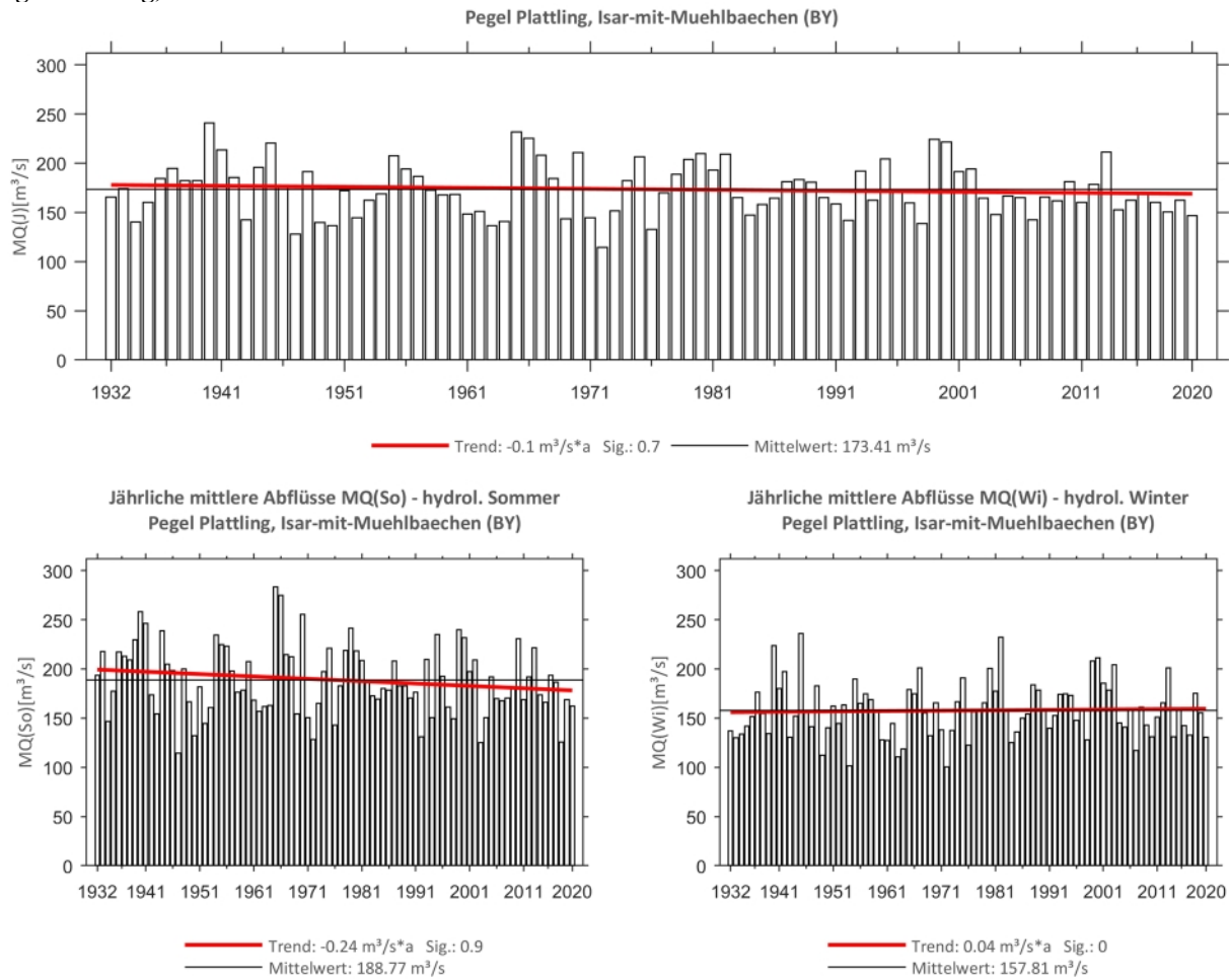
Abb. 126: Trenduntersuchungen von jährlichen mittleren Abflüssen für den Zeitraum 1932 bis 2020.
