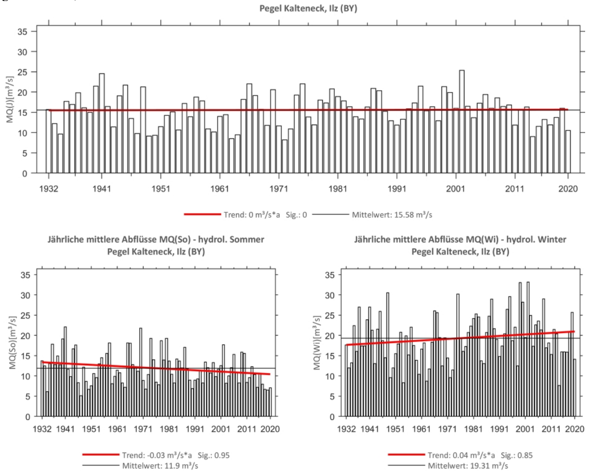
Abb. 72: Trenduntersuchungen von jährlichen mittleren Abflüssen für den Zeitraum 1932 bis 2020.
