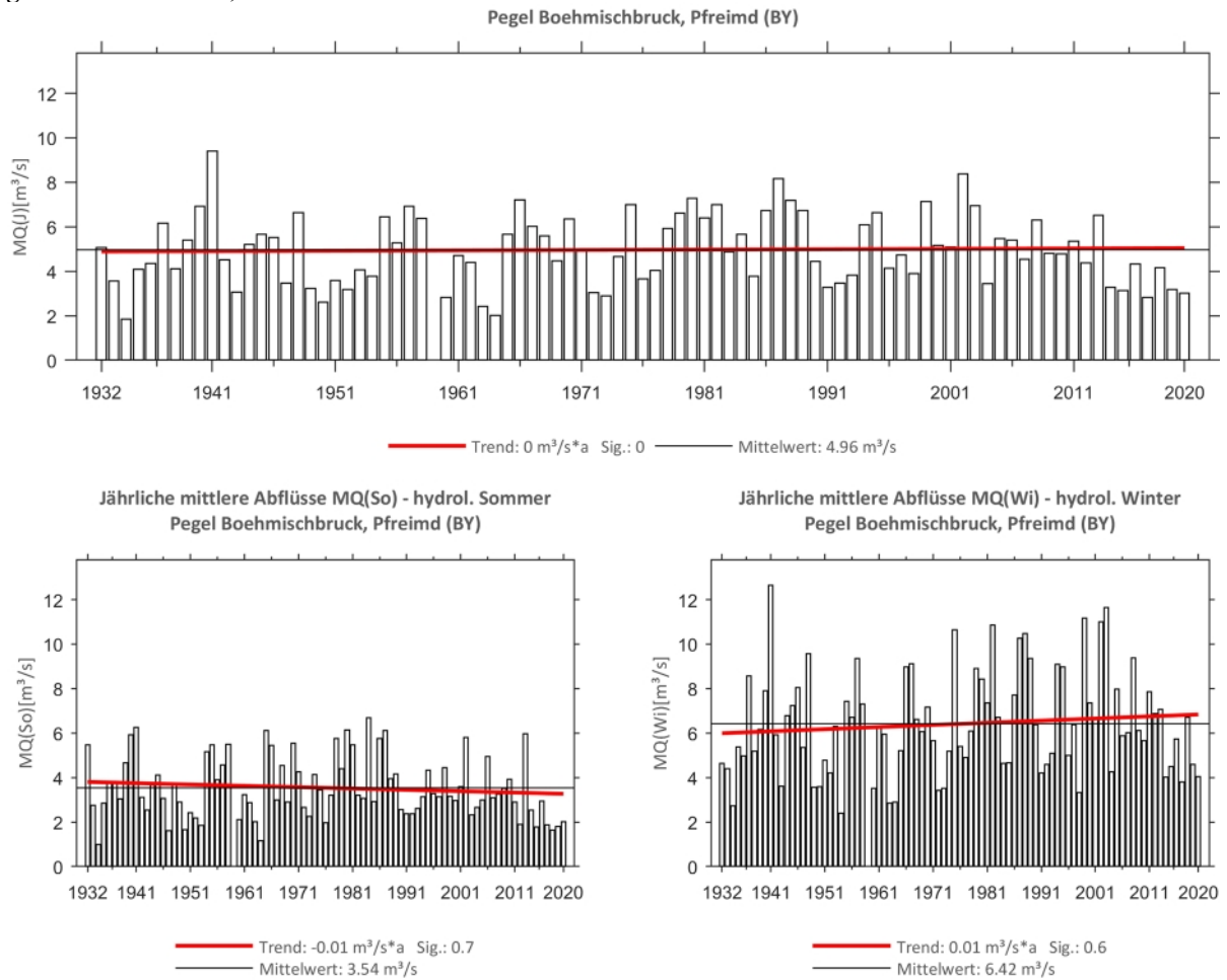
Abb. 64: Trenduntersuchungen von jährlichen mittleren Abflüssen für den Zeitraum 1932 bis 2020.
