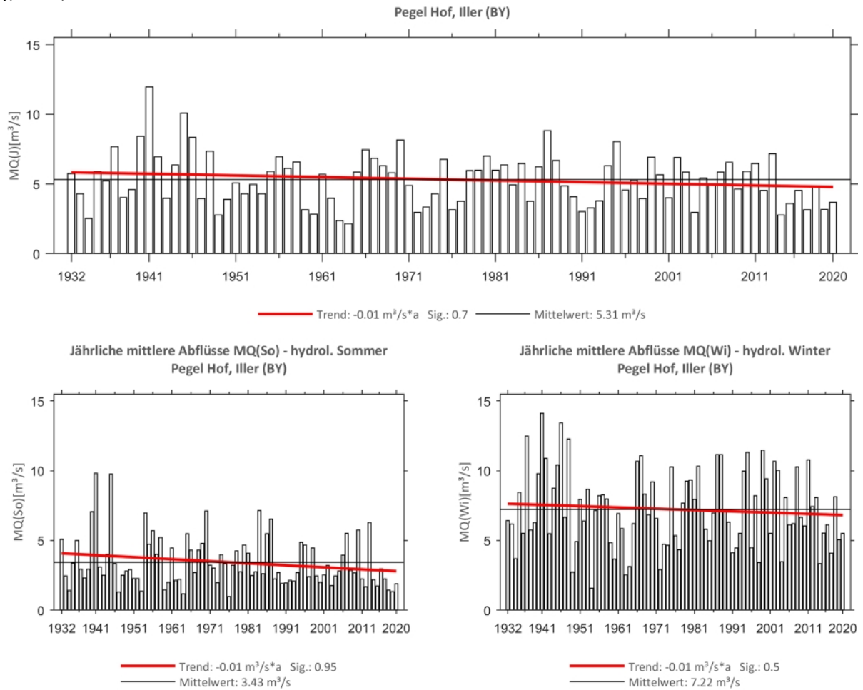
Abb. 68: Trenduntersuchungen von jährlichen mittleren Abflüssen für den Zeitraum 1932 bis 2020.
