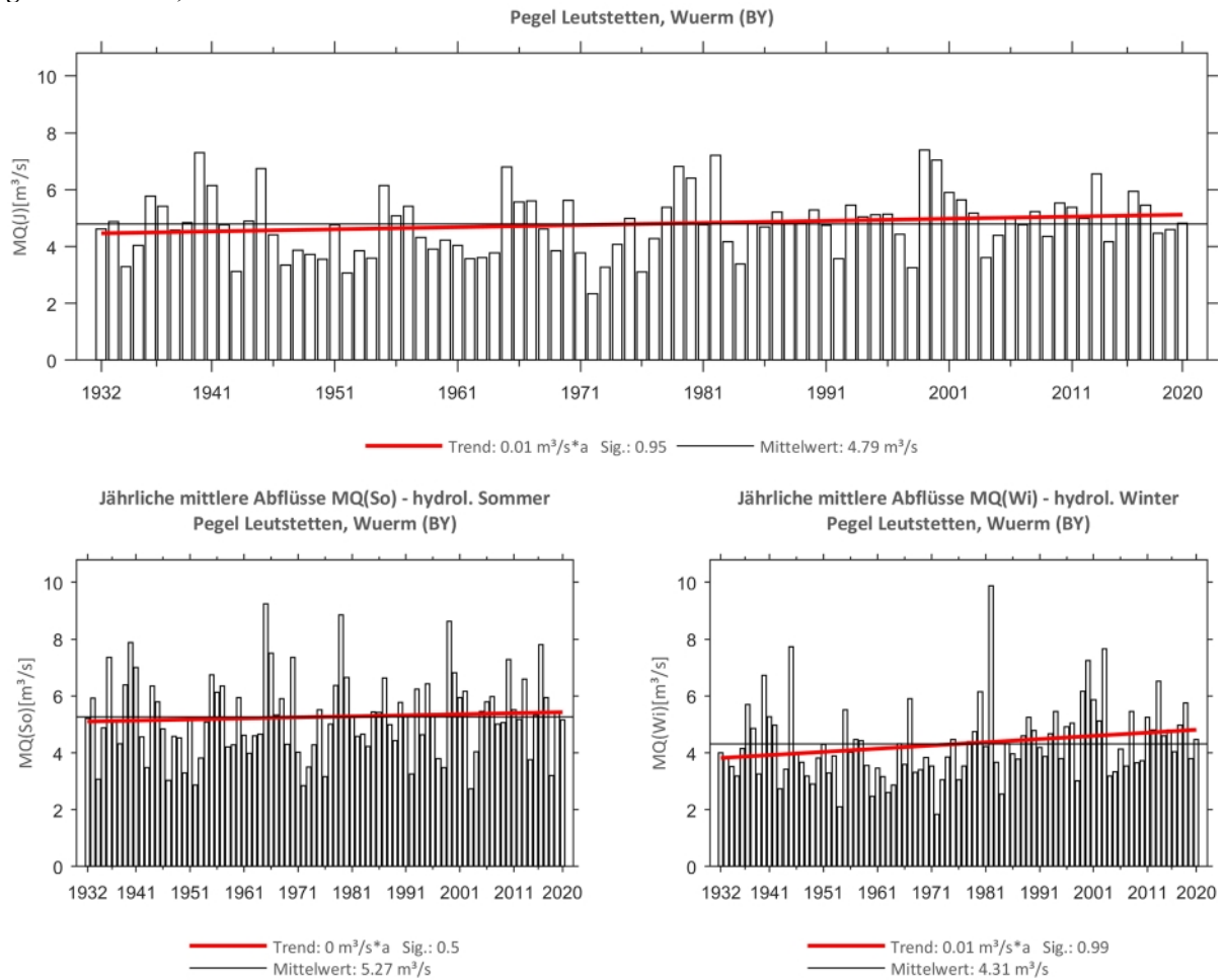
Abb. 116: Trenduntersuchungen von jährlichen mittleren Abflüssen für den Zeitraum 1932 bis 2020.
