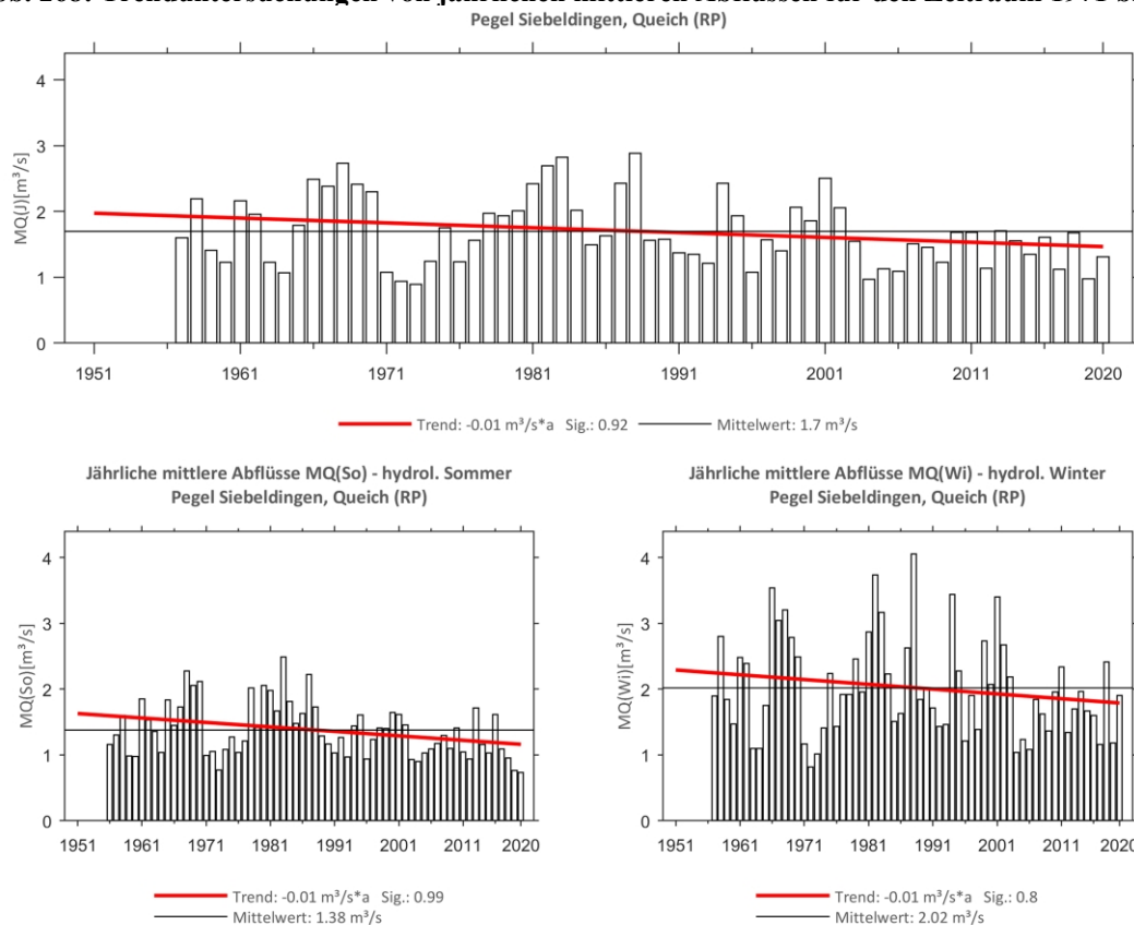
Abb. 269: Trenduntersuchungen von jährlichen mittleren Abflüssen für den Zeitraum 1957 bis 2020.
