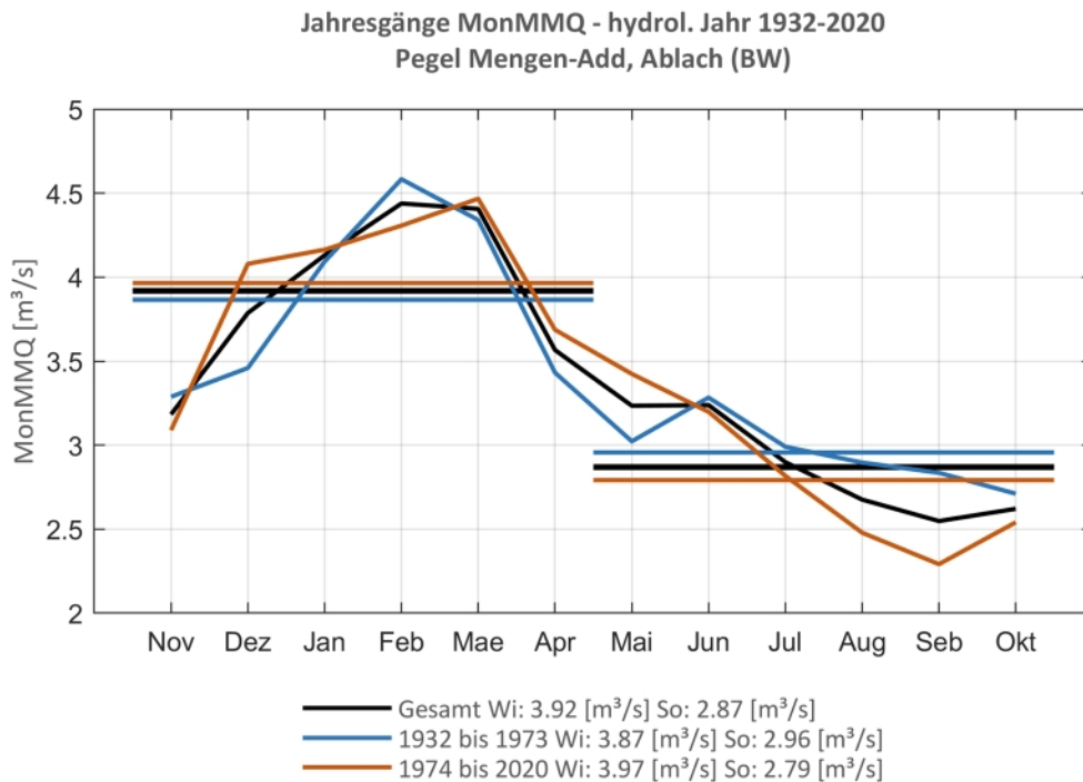
Abb. 59: Jahresgang des MonMMQ und Halbjahresmittel für 1932-2020 sowie 1932-1973 und 1974-2020.
