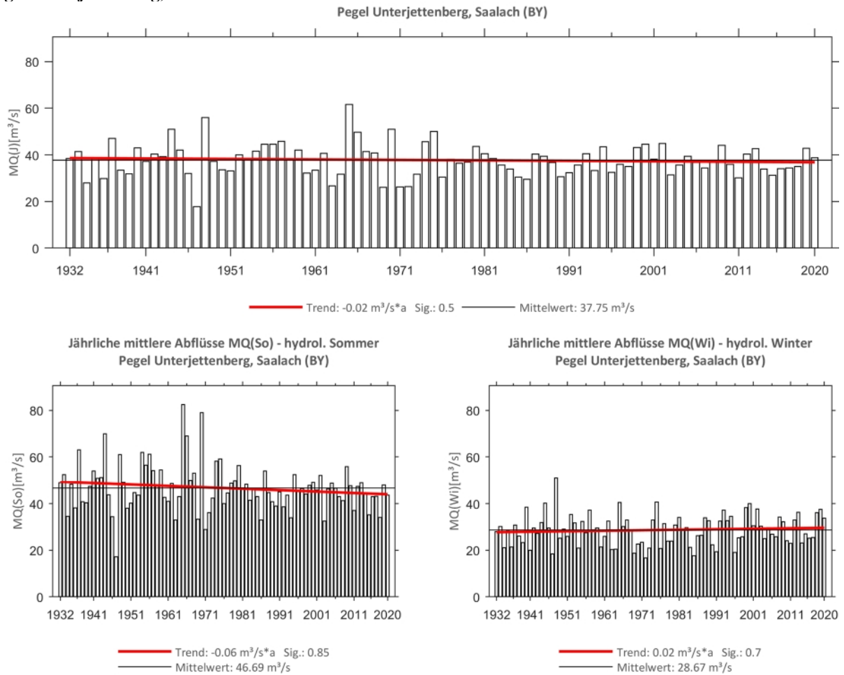
Abb. 136: Trenduntersuchungen von jährlichen mittleren Abflüssen für den Zeitraum 1932 bis 2020.
