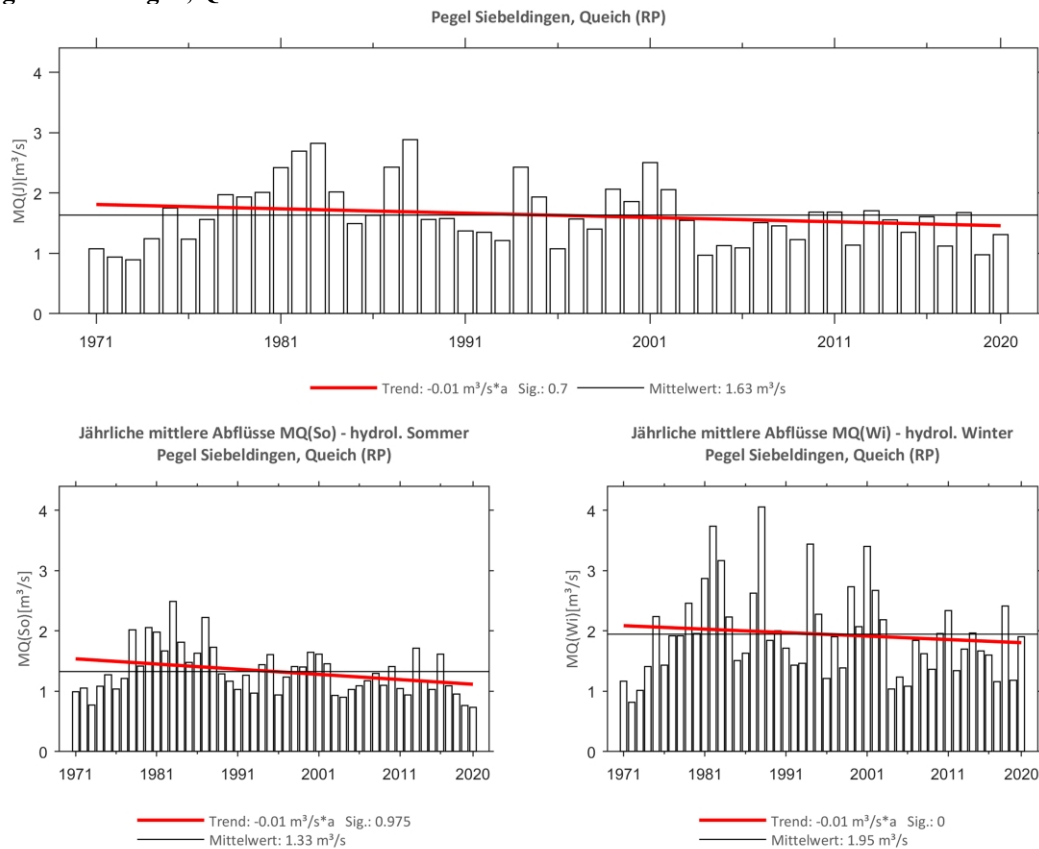
Abb. 268: Trenduntersuchungen von jährlichen mittleren Abflüssen für den Zeitraum 1971 bis 2020.
