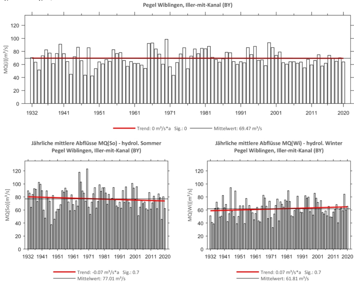
Abb. 94: Trenduntersuchungen von jährlichen mittleren Abflüssen für den Zeitraum 1932 bis 2020.
