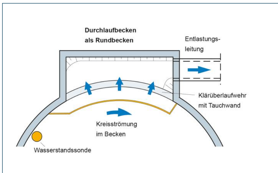
Abb. 31: Anordnung einer Wasserstandssonde in Rundbecken
