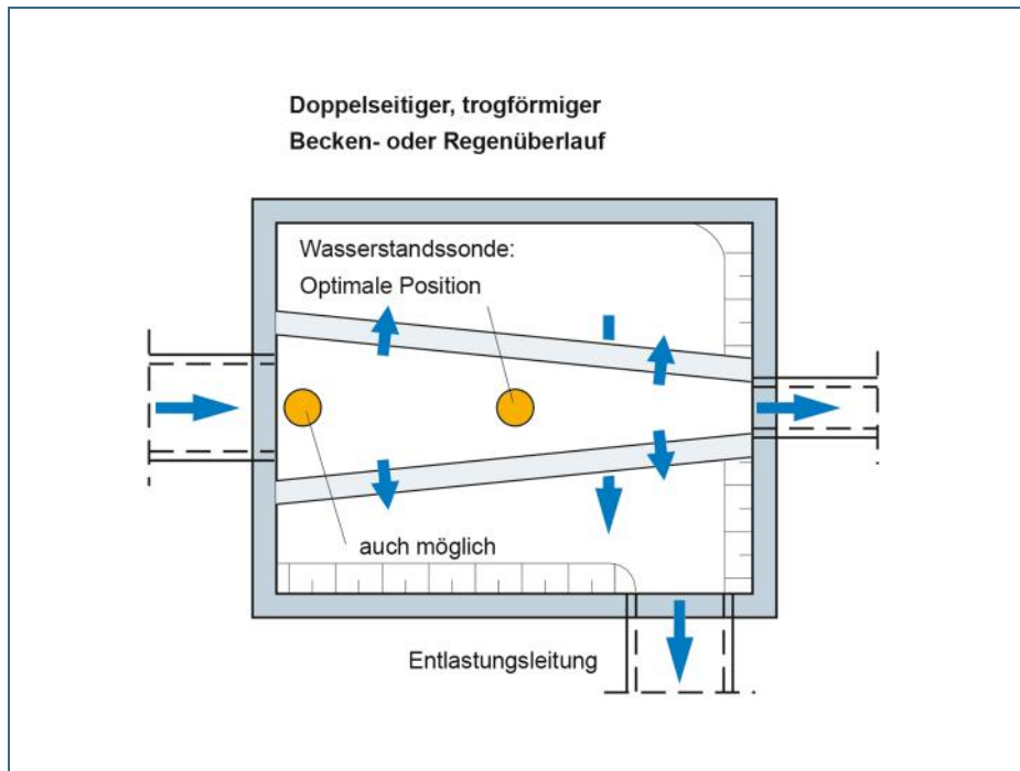
Abb. 30: Wasserstandsmessung in doppelseitigen Becken- oder Regen- überläufen
