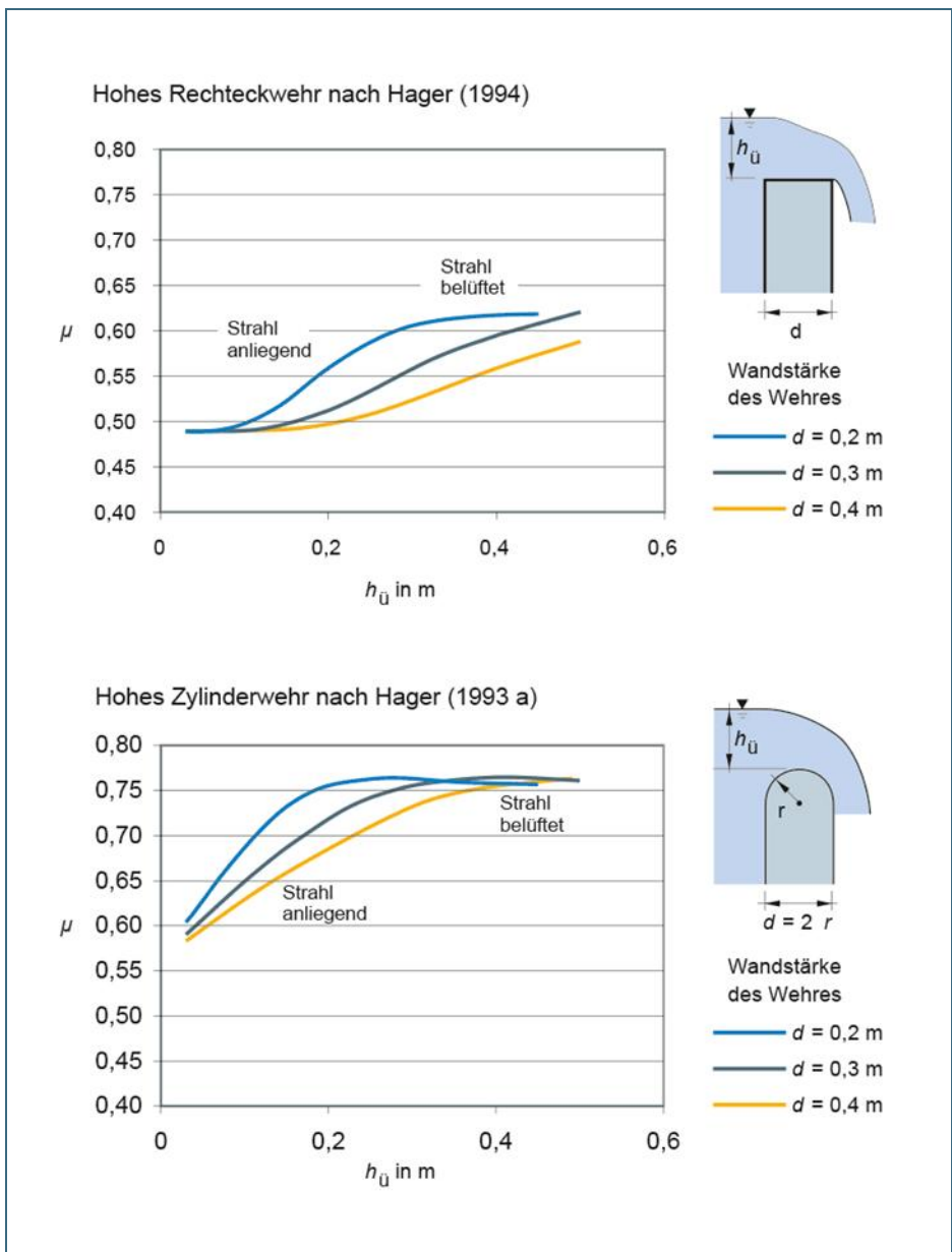
Abb. 17: Überfallbeiwerte \mu in Abhängigkeit von der Überfallhöhe h_u
