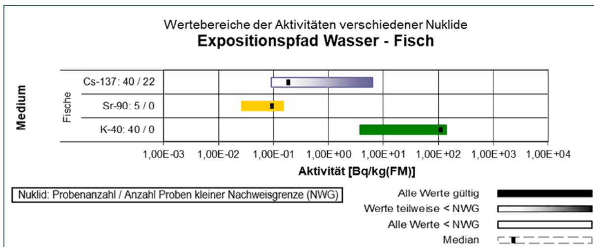
Abb. 3: Wertebereiche der in Bayern gemessenen Aktivitäten des Expositionspfads Ernährungskette Wasser im Jahr 2022
