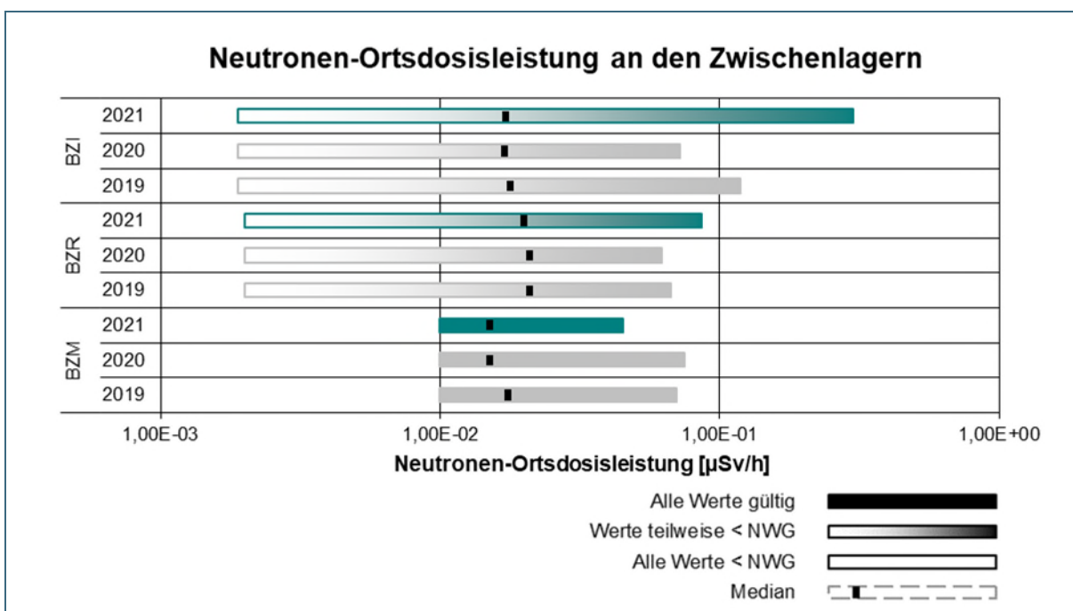
Abb. 12: Übersicht über die Wertebereiche der Neutronen-Ortsdosisleistung (N-ODL) an den Brennelement-zwischenlagern gem. REI, Tabelle C1.1, Punkt 1.3 im Jahr 2021 im Vergleich zu den Vorjahren 2020 und 2019
