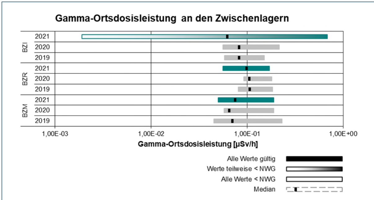
Abb. 11: Übersicht über die Wertebereiche der Gamma-Ortsdosisleistung (G-ODL) an den Brennelement-zwischenlagern gem. REI, Tabelle C1.1, Punkt 1.1 im Jahr 2021 im Vergleich zu den Vorjahren 2020 und 2019
