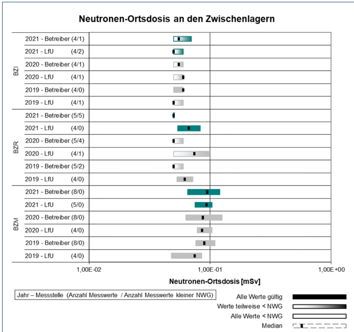
Abb. 14: Übersicht über die Wertebereiche der Neutronen-Ortsdosis (N-OD) an den Brennelementzwischenlagern gem. REI, Tabelle C.1.1, Punkt 1.4 und Tabelle C.1.2, Punkt 1.2 im Jahr 2021 im Vergleich zu den Vorjahren 2020 und 2019
