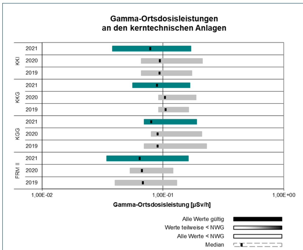
Abb. 9: Übersicht über die Wertebereiche der Gamma-Ortsdosisleistung an den kerntechnischen Anlagen (aus 10-Minuten-Messwerten) gem. REI, Tabelle A1, Punkt 1.1a im Jahr 2021 im Vergleich zu den Vorjahren 2020 und 2019
