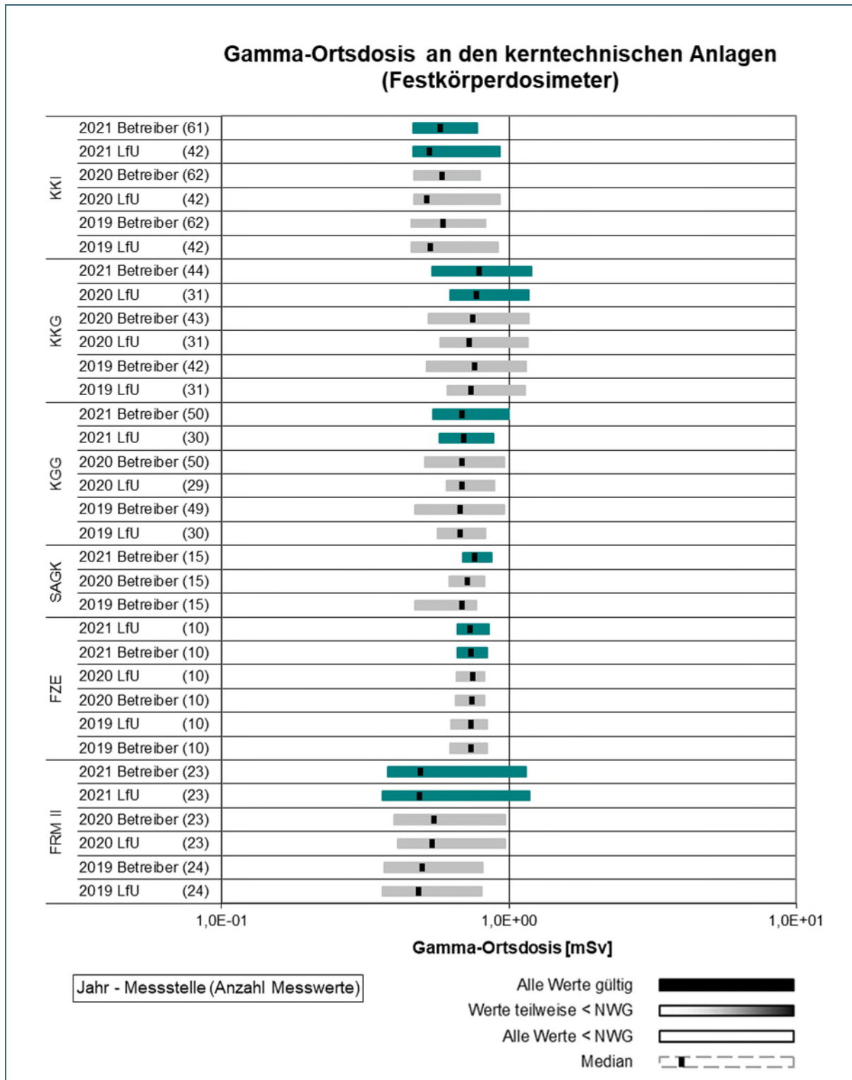
Abb. 10: Übersicht über die Wertebereiche der Gamma-Ortsdosis (Jahresdosis von Festkörperdosimetern) gem. REI, Tabelle A1, Punkt 1.1b und Tabelle A2, Punkt 1.1 im Jahr 2021 im Vergleich zu den Vorjahren 2020 und 2019
