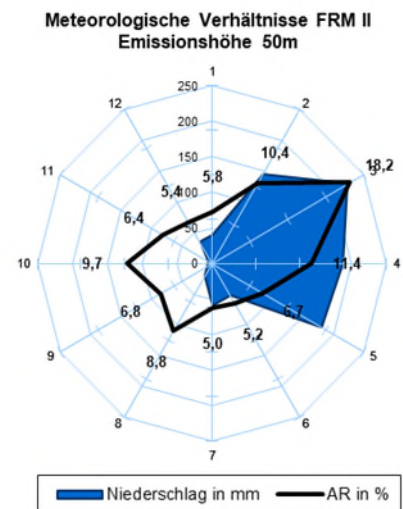
Abb. 15: Häufigkeitsverteilung der Ausbreitungsrichtung (AR) in % sowie die Niederschlagsmenge in mm pro Sektor der überwachten kerntechnischen Anlagen im Jahr 2021
