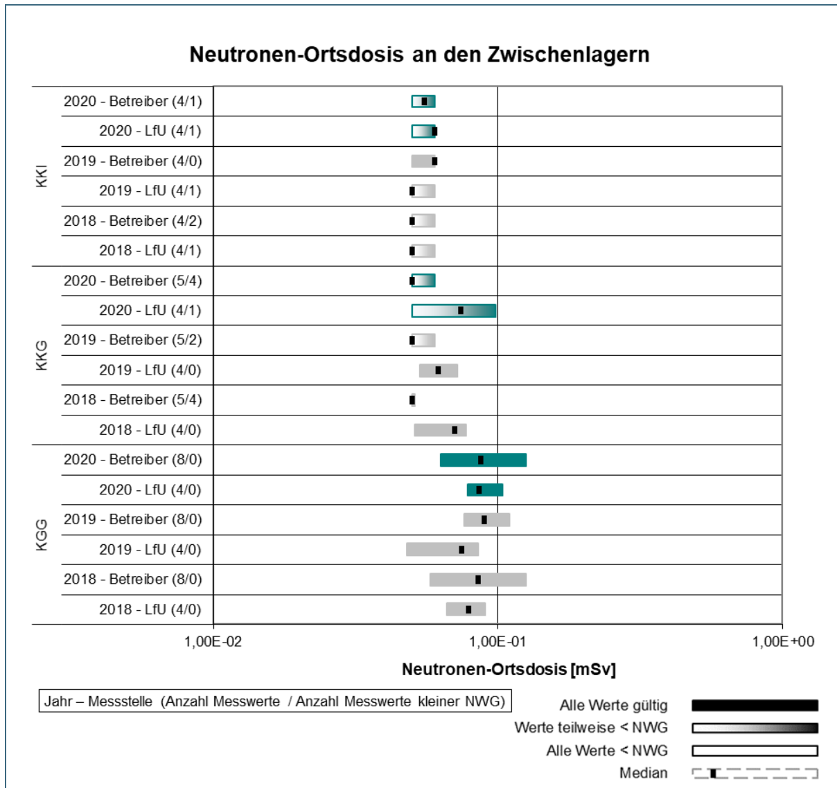
Abb. 14: Übersicht über die Wertebereiche der Neutronen-Ortsdosis (N-OD) an den Brennelementzwischenlagern gem. REI, Tabelle C.1.1, Punkt 1.4 und Tabelle C.1.2, Punkt 1.2 im Jahr 2020 im Vergleich zu den Vorjahren 2019 und 2018
