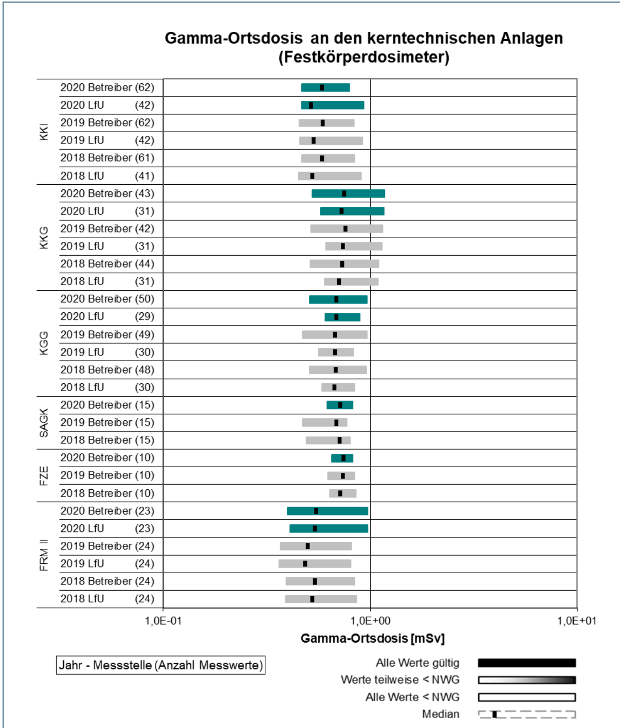
Abb. 10: Übersicht über die Wertebereiche der Gamma-Ortsdosis (Jahresdosis von Festkörperdosimetern) gem. REI, Tabelle A1, Punkt 1.1b und Tabelle A2, Punkt 1.1 im Jahr 2020 im Vergleich zu den Vorjahren 2019 und 2018
