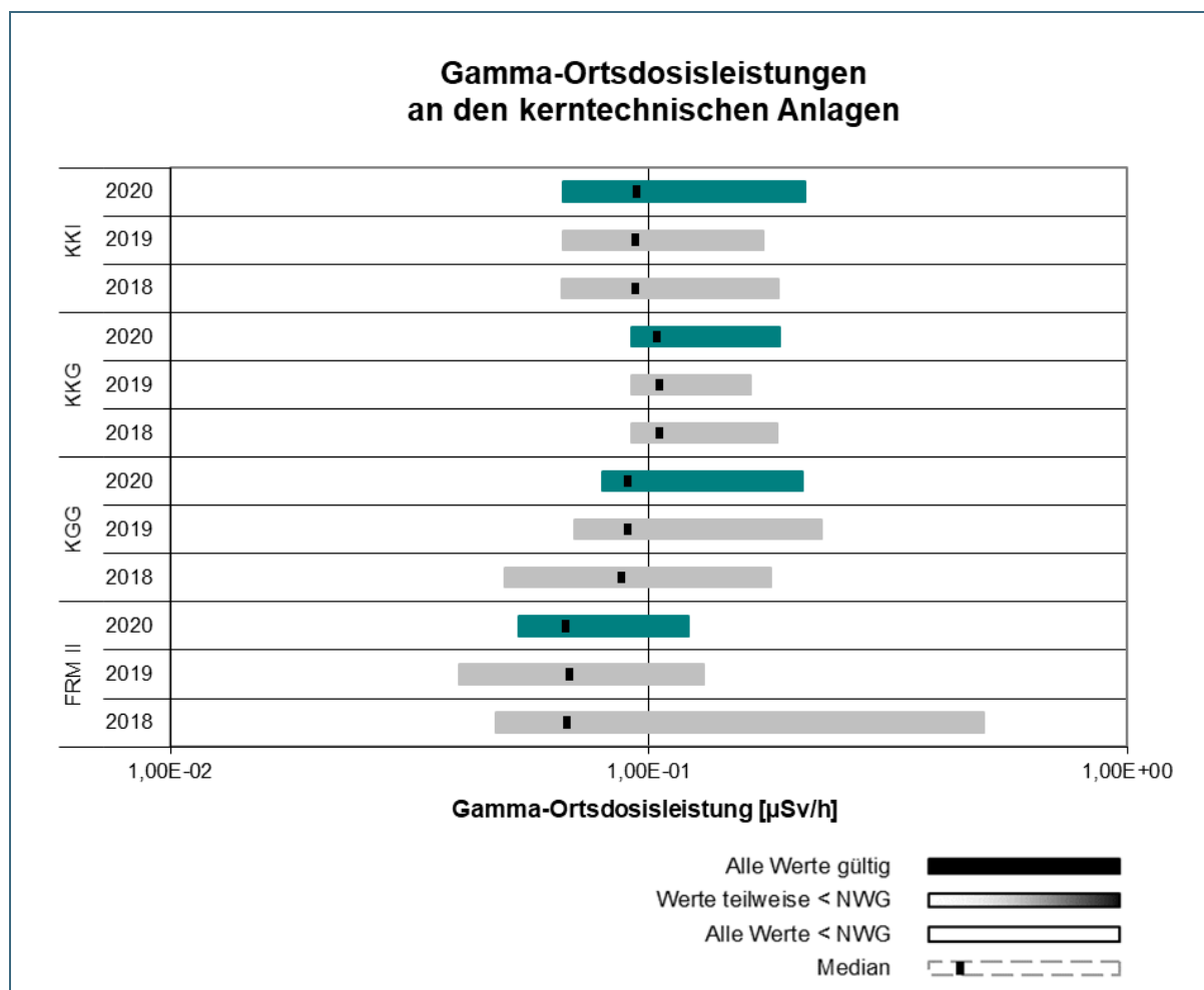
Abb. 9: Übersicht über die Wertebereiche der Gamma-Ortsdosisleistung an den kerntechnischen Anlagen (aus 10-Minuten-Messwerten) gem. REI, Tabelle A1, Punkt 1.1a im Jahr 2020 im Vergleich zu den Vorjahren 2019 und 2018
