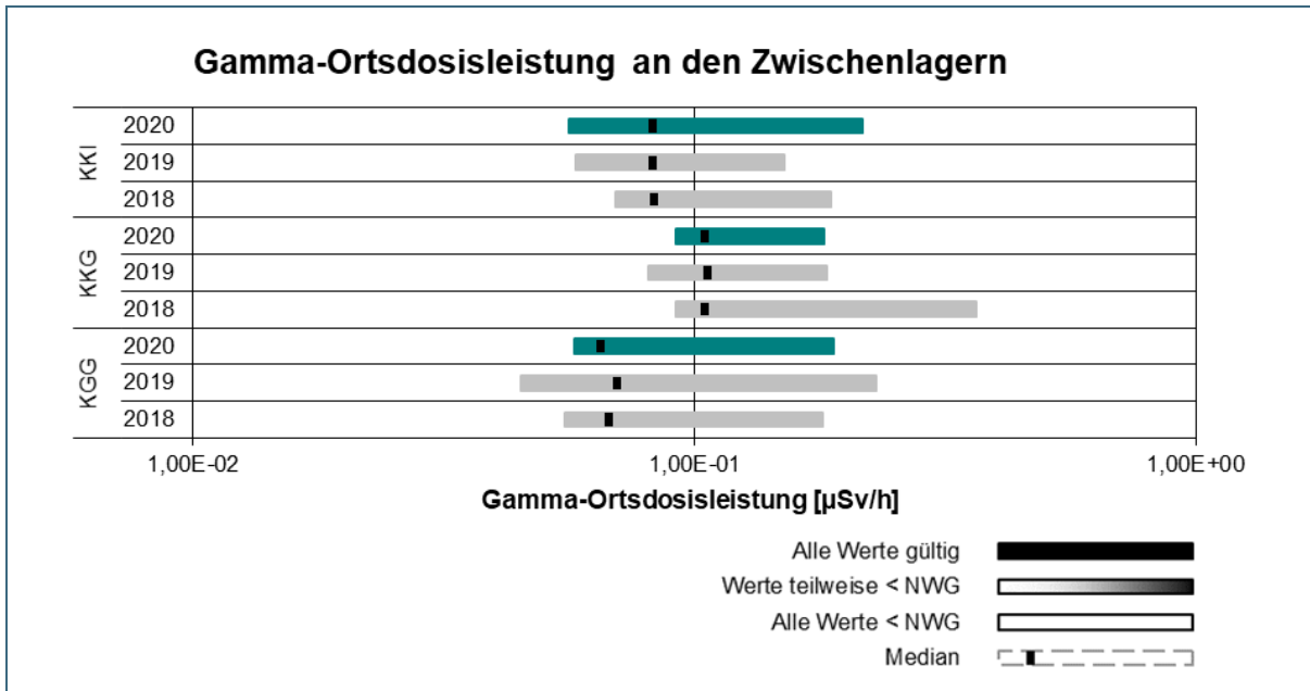
Abb. 11: Übersicht über die Wertebereiche der Gamma-Ortsdosisleistung (G-ODL) an den Brennelement-zwischenlagern gem. REI, Tabelle C1.1, Punkt 1.1 im Jahr 2020 im Vergleich zu den Vorjahren 2019 und 2018
