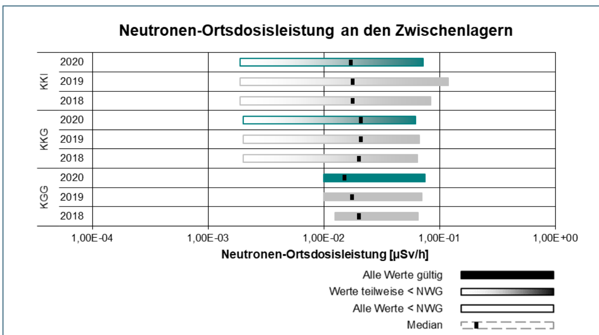
Abb. 12: Übersicht über die Wertebereiche der Neutronen-Ortsdosisleistung (N-ODL) an den Brennelement-zwischenlagern gem. REI, Tabelle C1.1, Punkt 1.3 im Jahr 2020 im Vergleich zu den Vorjahren 2019 und 2018
