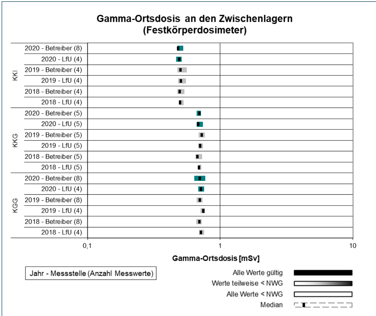
Abb. 13: Übersicht über die Wertebereiche der Gamma-Ortsdosis (G-OD) an den Brennelementzwischenlagern gem. REI, Tabelle C1.1, Punkt 1.2 und Tabelle C1.2, Punkt 1.1 im Jahr 2020 im Vergleich zu den Vorjahren 2019 und 2018
