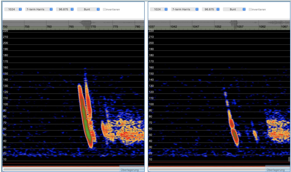
Abb. 1: Zwei Rufe aus der gleichen Sequenz einer „Bartfledermaus“ als Sonagramm mit den gleichen Einstellungen. Links: Bei guter Aufnahmequalität lassen sich die Rufparameter, wie Start- und Endfrequenz sicher bestimmen; Rechts: Der Ruf war zu leise, um mit gleich hoher Qualität aufgenommen werden zu können. Vermutlich hatte sich das Tier vom Mikrofon schon weiter entfernt oder hat in eine andere Richtung gerufen, sodass die Schallkeule am Mikrofon vorbeiging. Vor allem die Startfrequenz ist hier nicht mehr messbar, aber auch das Rufende ist wahrscheinlich unvollständig aufgezeichnet.
