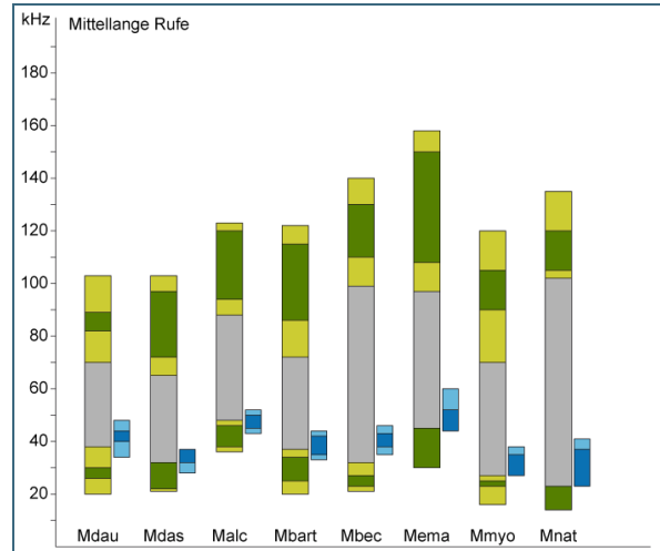
Abb. 45: Parameter mittellanger Rufe: Kernbereiche der Start- und Endfrequenzen in dunkelgrün, seltener auftretende Extremwerte in hellgrün; Kern- und Extremfrequenzbereiche des Myotisknicks in dunkel- und hellblau.
