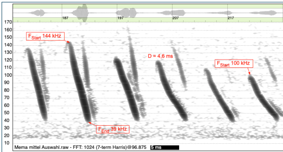
Abb. 32: Auswahl mittellanger, linear abfallender und leicht geschwungener Rufe der Wimperfledermaus (> 3,5–6 ms). Charakteristisch ist bei vielen Rufen ein Aufwärtsschwung am Rufanfang.
