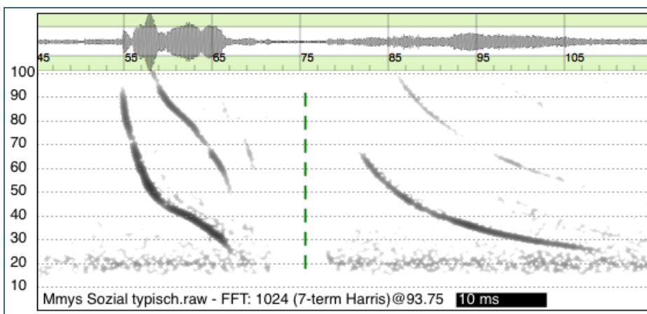
Abb. 24: Ortungsrufähnlicher Sozialruf (links) und Bogenruf (rechts) der Bartfledermaus
