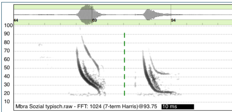
Abb. 23: Ortungsrufähnlicher Sozialruf (links) und Bogenruf (rechts) der Brandtfledermaus
