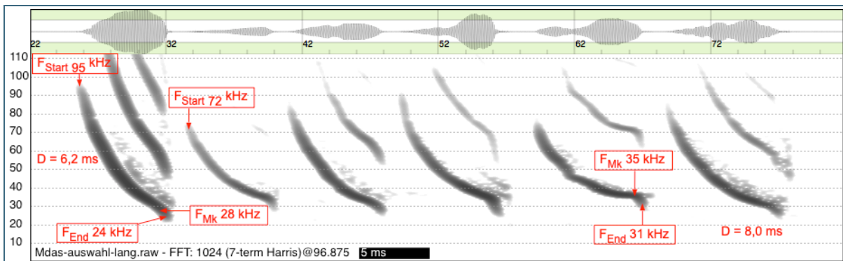
Abb. 10: Auswahl langer Rufe der Teichfledermaus (> 6–8 ms)
