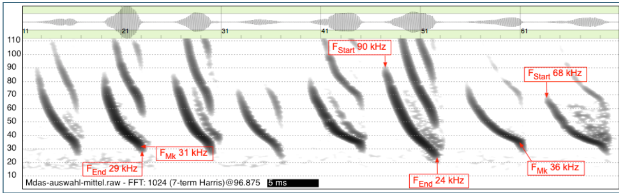
Abb. 9: Auswahl mittellanger Rufe der Teichfledermaus (> 3,5–6 ms)
