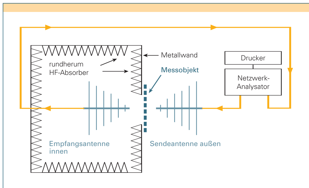
Abb. 7: Messanordnung zur Bestimmung der Schirmdämpfung (Prinzipiskizze)
