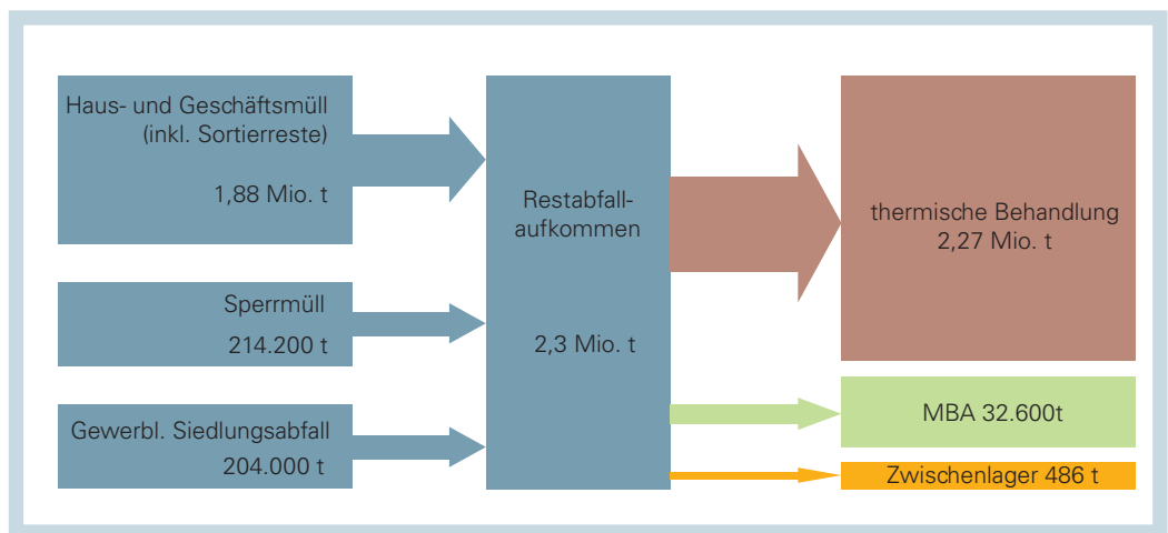
Abb. 13: Restabfallbehandlung in Bayern 2023
