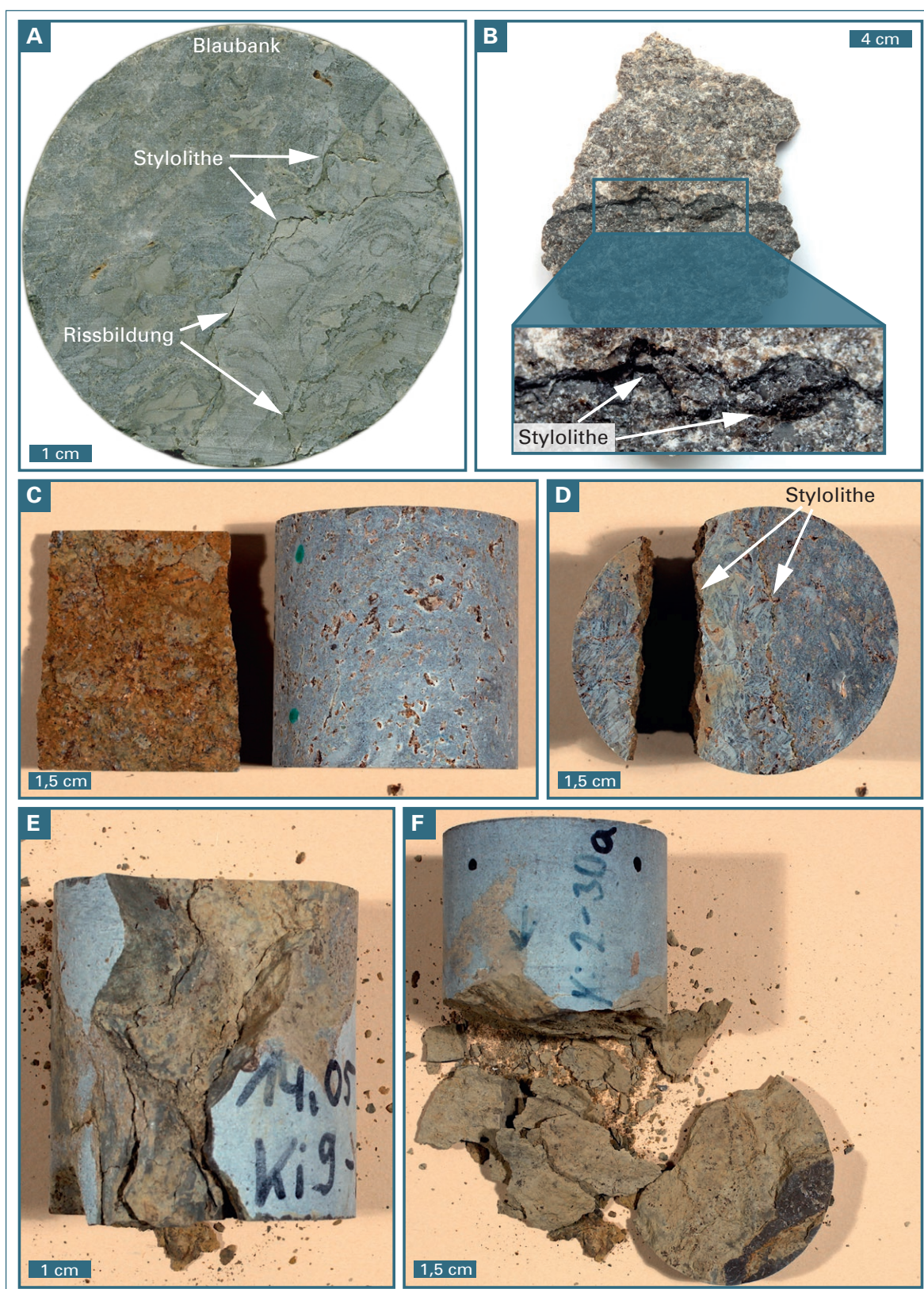
Abb. 40: Ausprägung und Verlauf verschiedener schadhafter Gefüge-Assoziationen innerhalb der untersuchten Prüfkörper. (A) Die Deckfläche eines Blaubank-Prüfkörpers mit Rissbildung entlang oder in der unmittelbaren Peripherie von zahlreichen kleinen Styrolithen (nach 168 FTW). (B) Nicht Frost-Tau-Wechsel beanspruchtes Handstück mit deutlich sichtbarem Styrolith. (C, D) Rotbank mit Riss an einem Styrolith. (E, F) Beschädigungen an Prüfkörpern aus der Messreihe der Gelbfaserkalkle.
