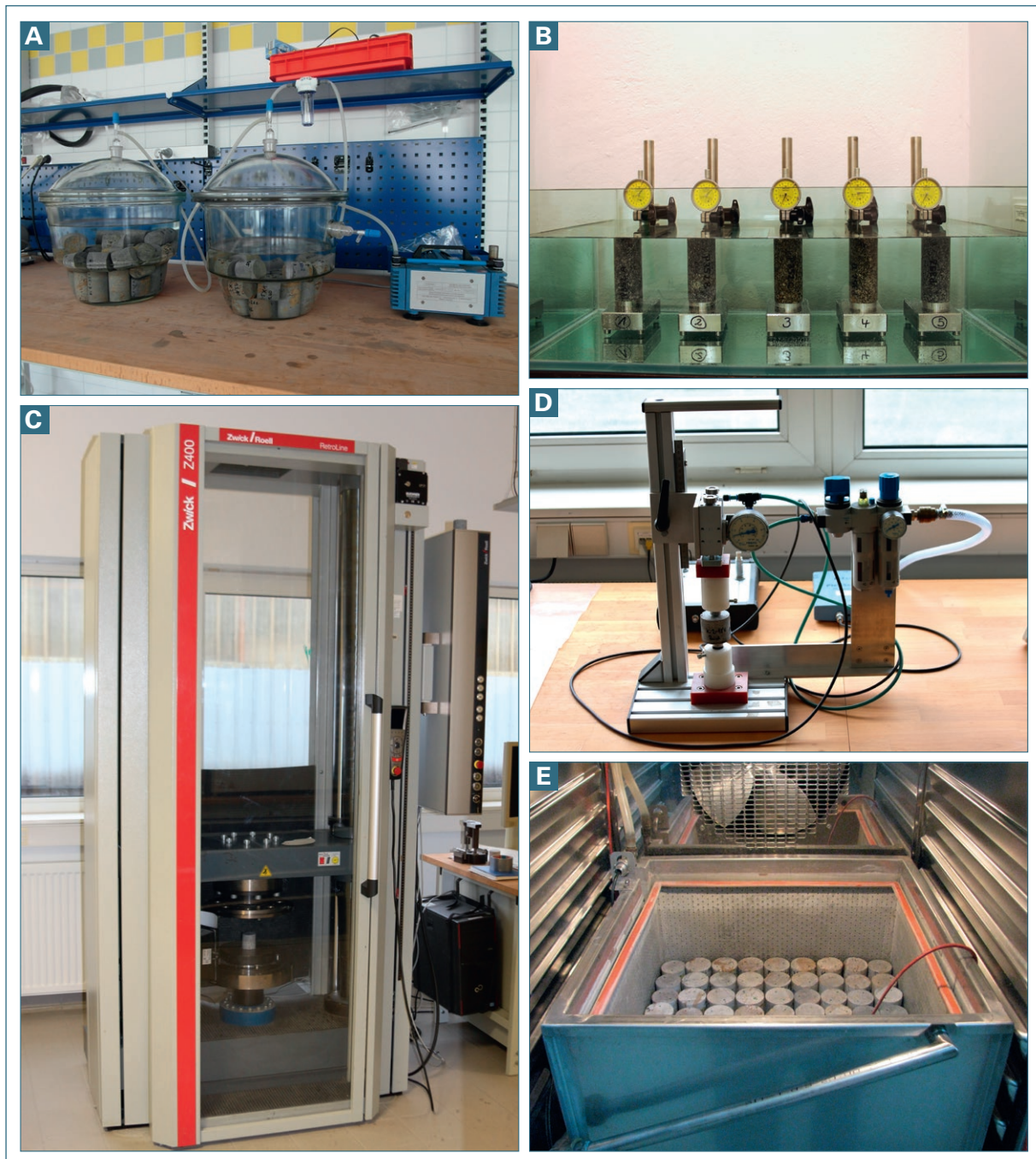
Abb. 9: Gesteinsphysikalische Versuchsdurchführung im Bohrkern- und Rohstoffanalytik-Zentrum in Hof. (A) Gesteinszylinder während der Wasseraufnahme unter Vakuum. (B) Versuchsanordnung zur Messung der hygrischen Dilatation mit Einspannvorrichtung, Messuhr und Prüfzylinder im Wasserbad. (C) Ermittlung der einaxialen Druckfestigkeit an der Universalprüfmaschine Z 400 der Fa. Zwick. (D) Messung der Kompressionswellengeschwindigkeit (Ultraschallprüfung). (E) Durchführung eines Frost-Tau-Wechsels in der Klimakammer.
