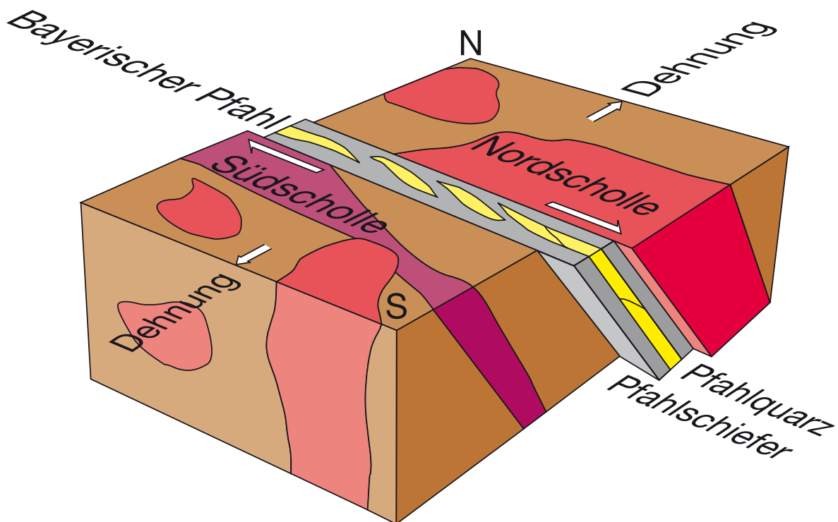
Schematische Darstellung der Bewegungen, die zum Aufreißen der Fiederspaltengänge führten, in denen sich der Pfahlquarz abscheiden konnte
