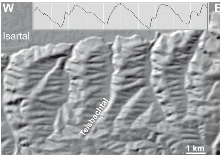
Geländerelevanz und überhöhter Schnitt im Bereich des Teisbachtals (Datengrundlage: Bayerisches Landesvermessungsamt)
