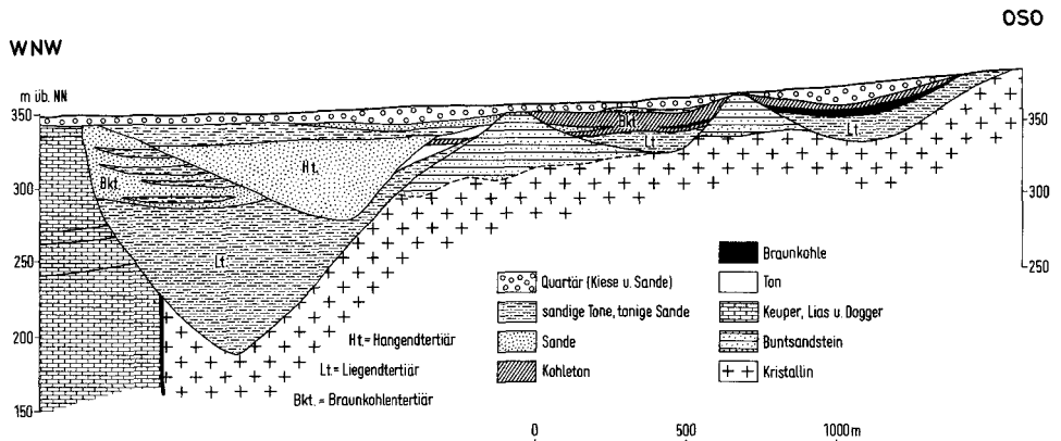
Abb. 6 Geologischer Querschnitt durch das Naabtertiär bei Teublitz (vereinfacht nach H. TILLMANN 1956)
