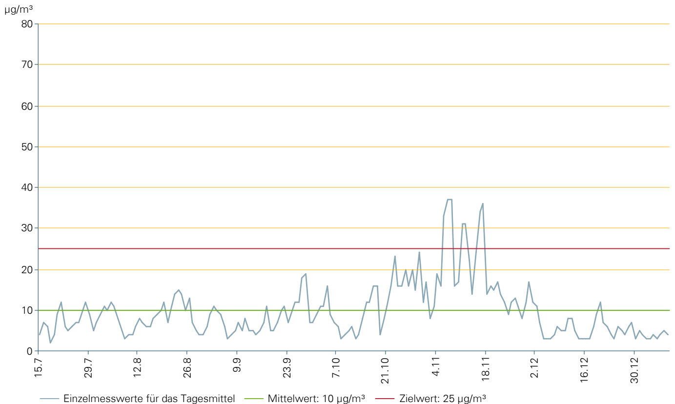
Verlauf der Feinstaub-Konzentration über den Messzeitraum vom 15. Juli 2011 bis 08. Januar 2012: Einzelmesswerte für das Tagesmittel, der Mittelwert und der Zielwert über den gesamten Messzeitraum
