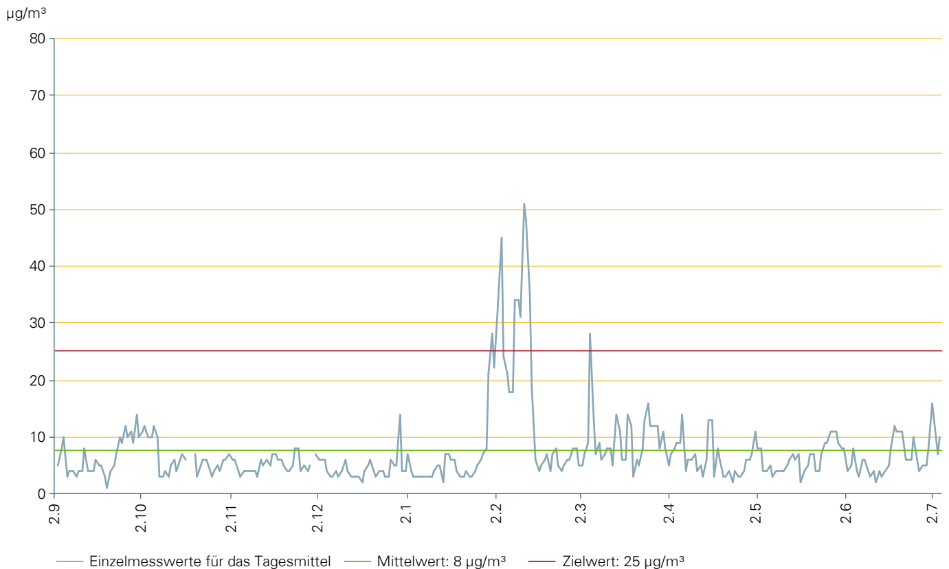
Verlauf der Feinstaub-Konzentration über den Messzeitraum vom 02. September 2011 bis 04. Juli 2012: Einzelmesswerte für das Tagesmittel, der Mittelwert und der Zielwert über den gesamten Messzeitraum
