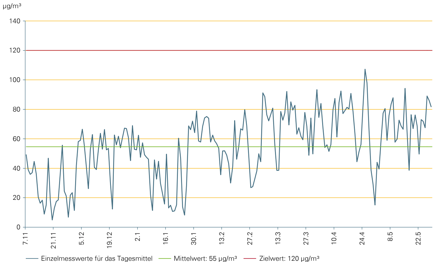
Verlauf der Ozon-Konzentration über den Messzeitraum vom 7. November 2012 bis 28. Mai 2013: Einzelmesswerte für das Tagesmittel, der Mittelwert und der Zielwert über den gesamten Messzeitraum
