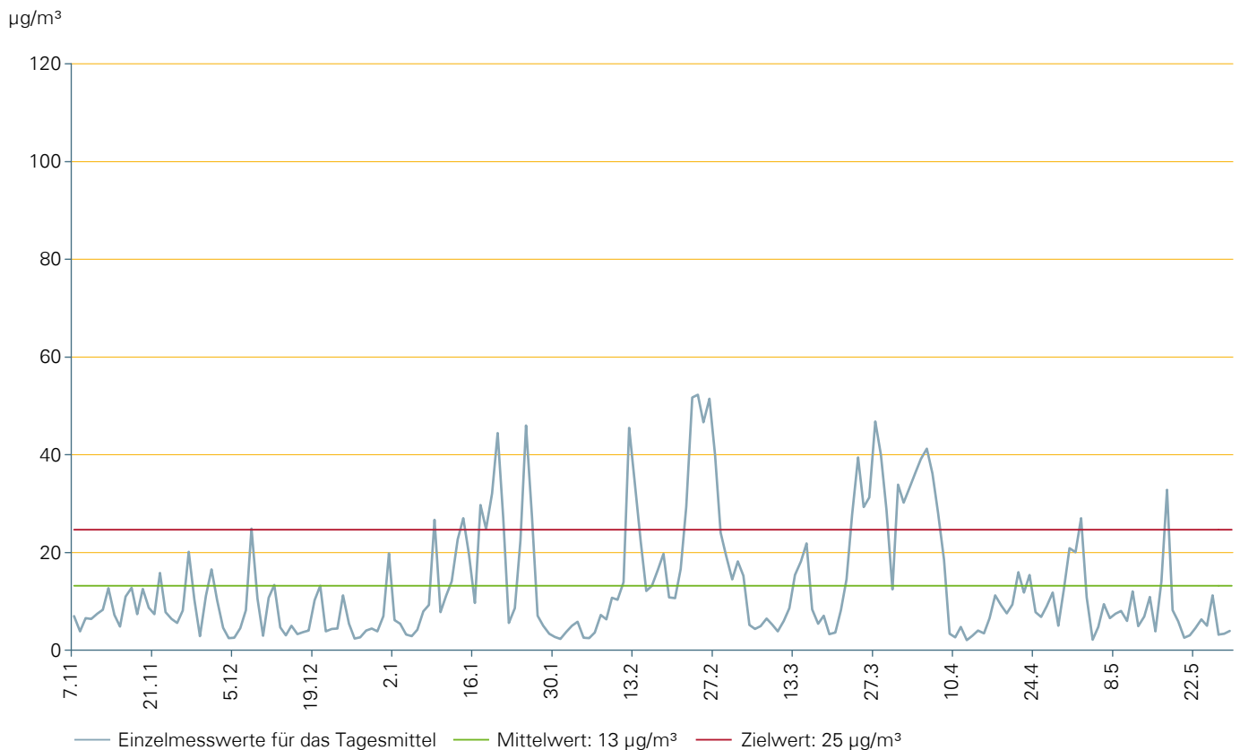
Verlauf der Feinstaub-Konzentration über den Messzeitraum vom 7. November 2012 bis 28. Mai 2013: Einzelmesswerte für das Tagesmittel, der Mittelwert und der Zielwert über den gesamten Messzeitraum
