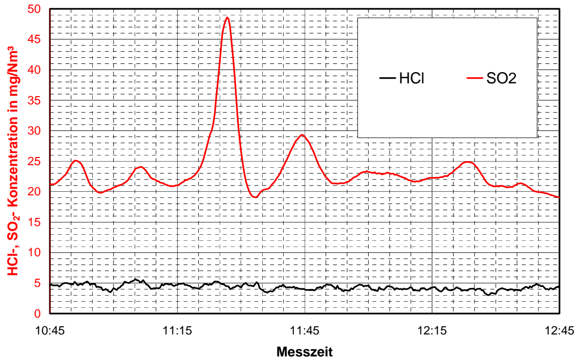
Bild 6.10-4: Zeitlicher Verlauf der HCl- und SO 2 - Konzentrationen bei voller Leistung der Kesselanlage
